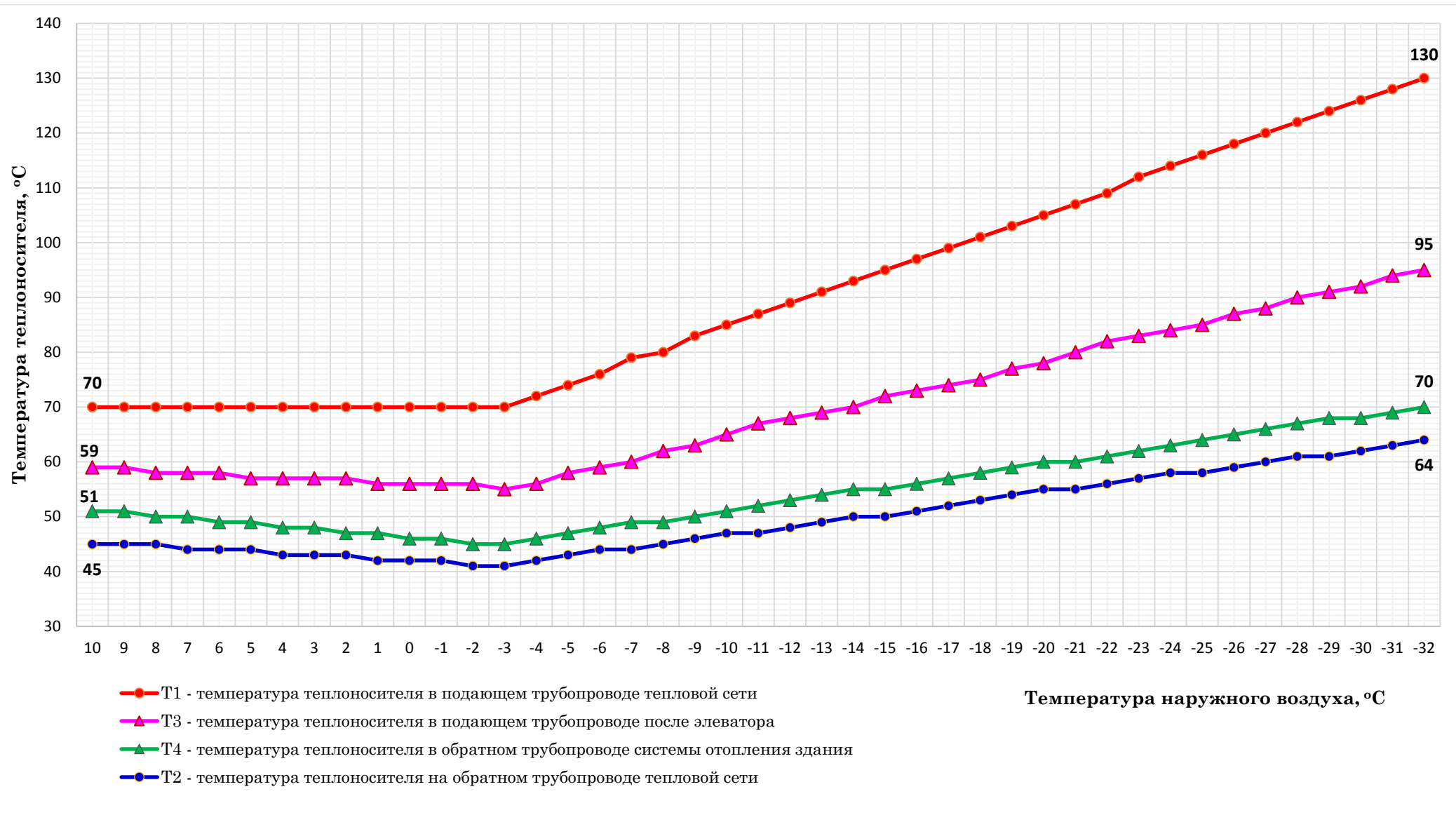
Рисунок 5.1 График температурного регулирования отпуска тепловой энергии 130/70 °C от котельной на ул. Умбо-зерская, д. 6 п.г.т. Ревда АО «МЭС»
